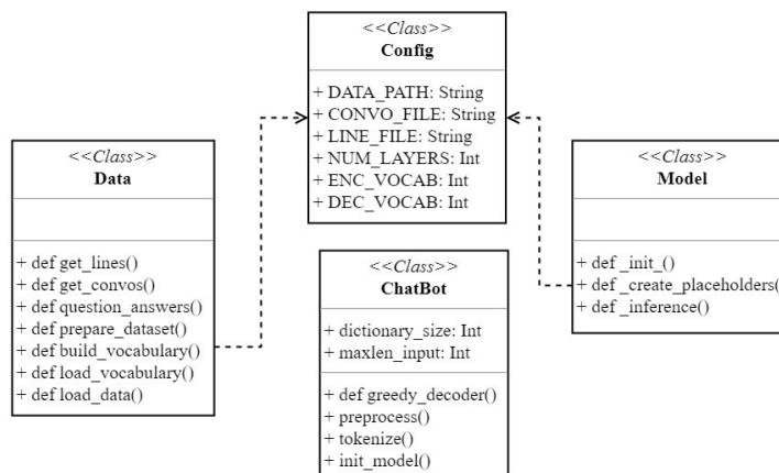
Рисунок 10. Діаграма класів прототипу інтелектуального чат-боту
